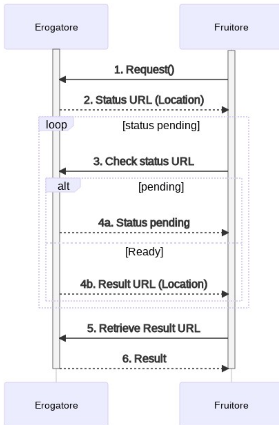
Figura 3 - Interazione non bloccante tramite busy waiting REST
