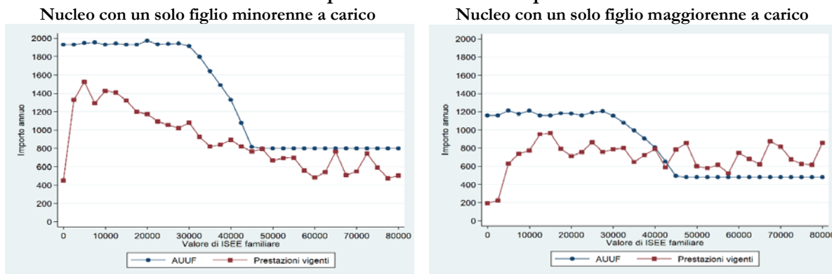
Figura A1. Assegno annuo con importo variabile e Prestazioni vigenti lungo la distribuzione ISEE per due casi familiari tipici
