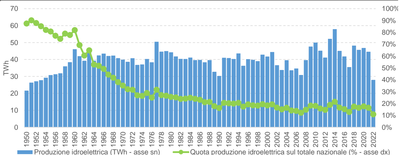
Graf. 2 – Evoluzione della produzione idroelettrica in Italia
