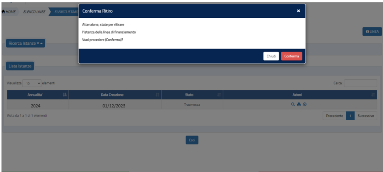
Figura 35 - Conferma Ritiro
