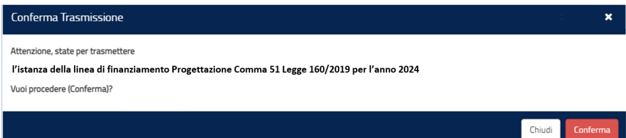
Figura 29 - Conferma Trasmissione
