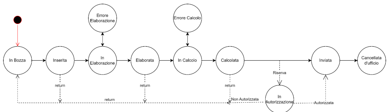
Figura 1 - Stati Processo Applicativo Qualificazione Stazioni Appaltanti
