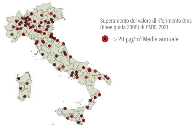
Figura 24: superamento del valore di riferimento Oms (linee guida 2005) di PM10 e PM2,5 9 rilevato tra tutte le centraline fisse per il monitoraggio della qualità dell'aria, per comune capoluogo di provincia/città metropolitana 3 . Anno 2021.
